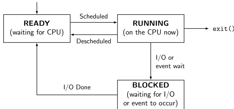
Figura 4.1: Diagramma a tre stati del ciclo di vita di un processo
